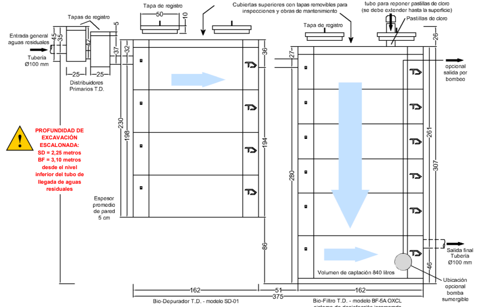
SISTEMA DE TRATAMIENTO TANQUE DIEZ MODELO PTB-OX80 - CAUDAL DIARIO A TRATAR 8 M 3 VISTA VERTICAL DE LAS UNIDADES DE TRATAMIENTO - MEDIDAS EN CENTÍMETROS TANQUE DIEZ - DERECHOS RESERVADOS
