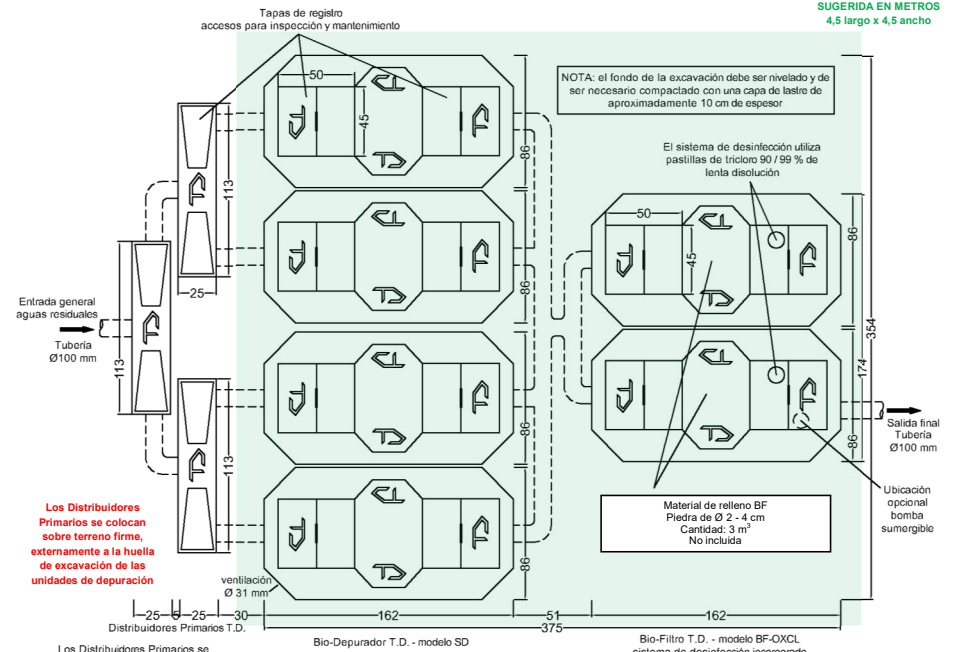
SISTEMA DE TRATAMIENTO TANQUE DIEZ MODELO PTB-OX80 - CAUDAL DIARIO A TRATAR 8 M 3 VISTA SUPERIOR DE LAS UNIDADES DE TRATAMIENTO - MEDIDAS EN CENTÍMETROS TANQUE DIEZ - DERECHOS RESERVADOS
