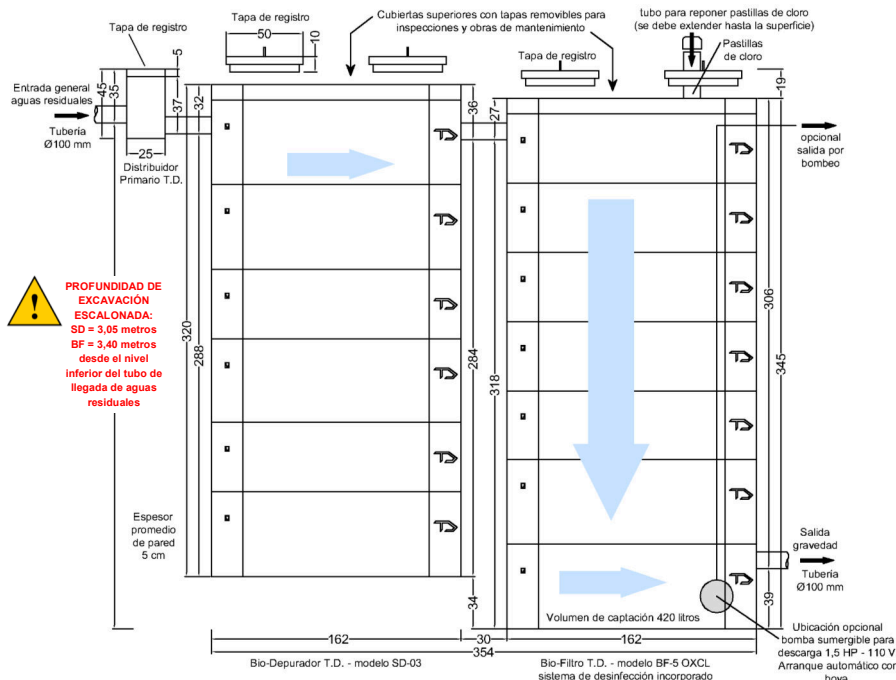
SISTEMA DE TRATAMIENTO TANQUE DIEZ MODELO PTB-OX60 - CAUDAL DIARIO A TRATAR 6 M 3 VISTA VERTICAL DE LAS UNIDADES DE TRATAMIENTO - MEDIDAS EN CENTÍMETROS TANQUE DIEZ - DERECHOS RESERVADOS
