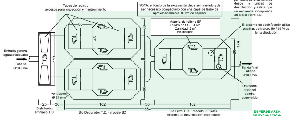
SISTEMA DE TRATAMIENTO TANQUE DIEZ MODELO PTB-OX60 - CAUDAL DIARIO A TRATAR 6 M 3 VISTA SUPERIOR DE LAS UNIDADES DE TRATAMIENTO - MEDIDAS EN CENTÍMETROS TANQUE DIEZ - DERECHOS RESERVADOS
