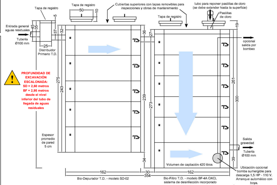
SISTEMA DE TRATAMIENTO TANQUE DIEZ MODELO PTB-OX50 - CAUDAL DIARIO A TRATAR 5 M 3 VISTA VERTICAL DE LAS UNIDADES DE TRATAMIENTO - MEDIDAS EN CENTÍMETROS TANQUE DIEZ - DERECHOS RESERVADOS
