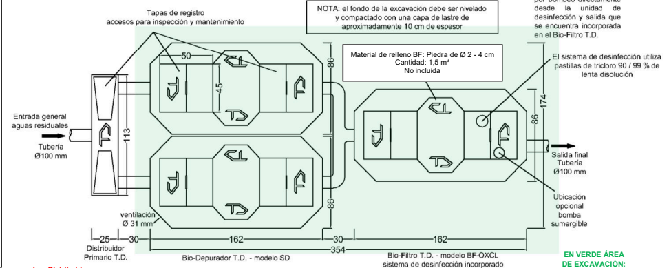
SISTEMA DE TRATAMIENTO TANQUE DIEZ MODELO PTB-OX50 - CAUDAL DIARIO A TRATAR 5 M 3 VISTA SUPERIOR DE LAS UNIDADES DE TRATAMIENTO - MEDIDAS EN CENTÍMETROS TANQUE DIEZ - DERECHOS RESERVADOS
