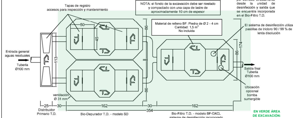
SISTEMA DE TRATAMIENTO TANQUE DIEZ MODELO PTB-OX40 - CAUDAL DIARIO A TRATAR 4 M 3 VISTA SUPERIOR DE LAS UNIDADES DE TRATAMIENTO - MEDIDAS EN CENTÍMETROS TANQUE DIEZ - DERECHOS RESERVADOS
