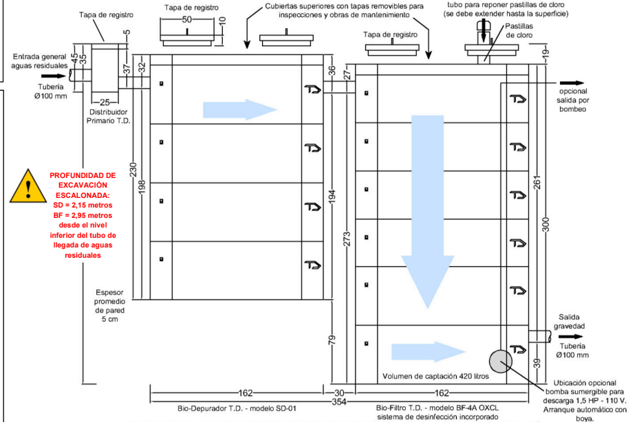
SISTEMA DE TRATAMIENTO TANQUE DIEZ MODELO PTB-OX40 - CAUDAL DIARIO A TRATAR 4 M 3 VISTA VERTICAL DE LAS UNIDADES DE TRATAMIENTO - MEDIDAS EN CENTÍMETROS TANQUE DIEZ - DERECHOS RESERVADOS
