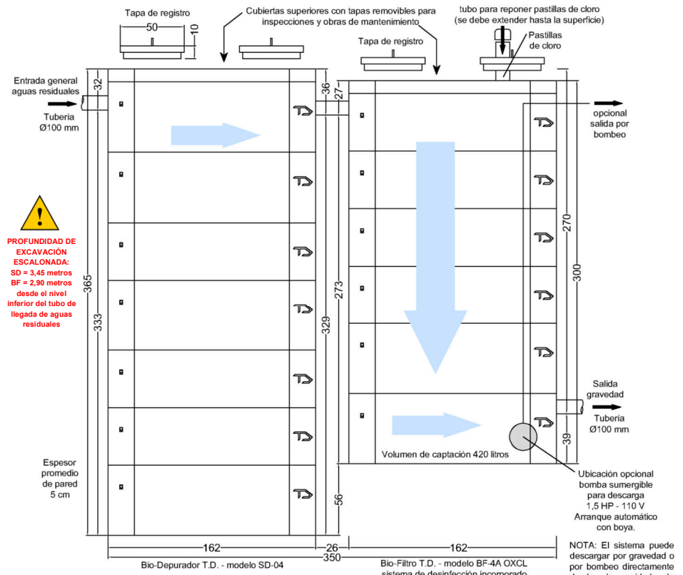
SISTEMA DE TRATAMIENTO TANQUE DIEZ MODELO PTB-OX35 - CAUDAL DIARIO A TRATAR 3,5 M 3 VISTA VERTICAL DE LAS UNIDADES DE TRATAMIENTO - MEDIDAS EN CENTIMETROS TANQUE DIEZ - DERECHOS RESERVADOS
