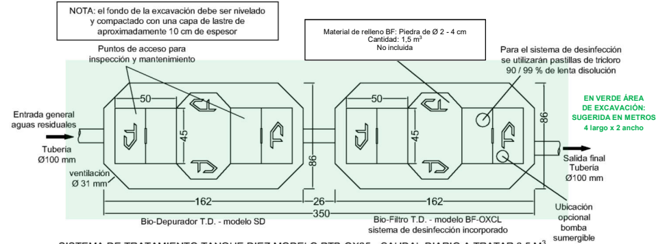
SISTEMA DE TRATAMIENTO TANQUE DIEZ MODELO PTB-OX35 - CAUDAL DIARIO A TRATAR 3,5 M 3 VISTA SUPERIOR DE LAS UNIDADES DE TRATAMIENTO - MEDIDAS EN CENTIMETROS TANQUE DIEZ - DERECHOS RESERVADOS
