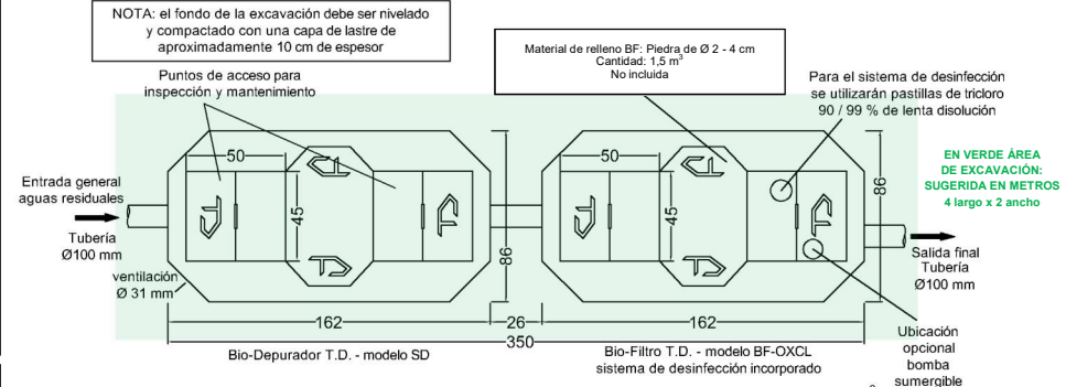
SISTEMA DE TRATAMIENTO TANQUE DIEZ MODELO PTB-OX30 - CAUDAL DIARIO A TRATAR 3 M 3 VISTA SUPERIOR DE LAS UNIDADES DE TRATAMIENTO - MEDIDAS EN CENTÍMETROS TANQUE DIEZ - DERECHOS RESERVADOS
