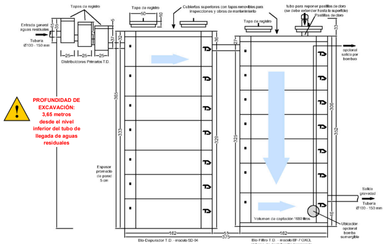
SISTEMA DE TRATAMIENTO TANQUE DIEZ MODELO PTB-OX280 - CAUDAL DIARIO A TRATAR 28 M 3 VISTA VERTICAL DE LAS UNIDADES DE TRATAMIENTO - MEDIDAS EN CENTIMETROS TANQUE DIEZ - DERECHOS RESERVADOS
