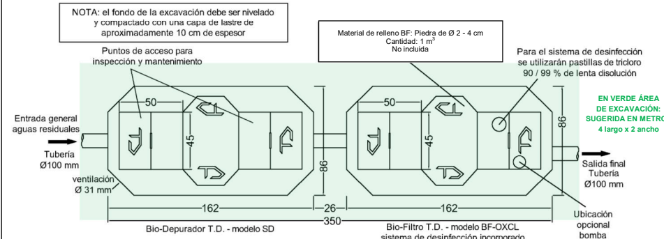
SISTEMA DE TRATAMIENTO TANQUE DIEZ MODELO PTB-OX25 - CAUDAL DIARIO A TRATAR 2,5 M 3 VISTA SUPERIOR DE LAS UNIDADES DE TRATAMIENTO - MEDIDAS EN CENTÍMETROS TANQUE DIEZ - DERECHOS RESERVADOS
