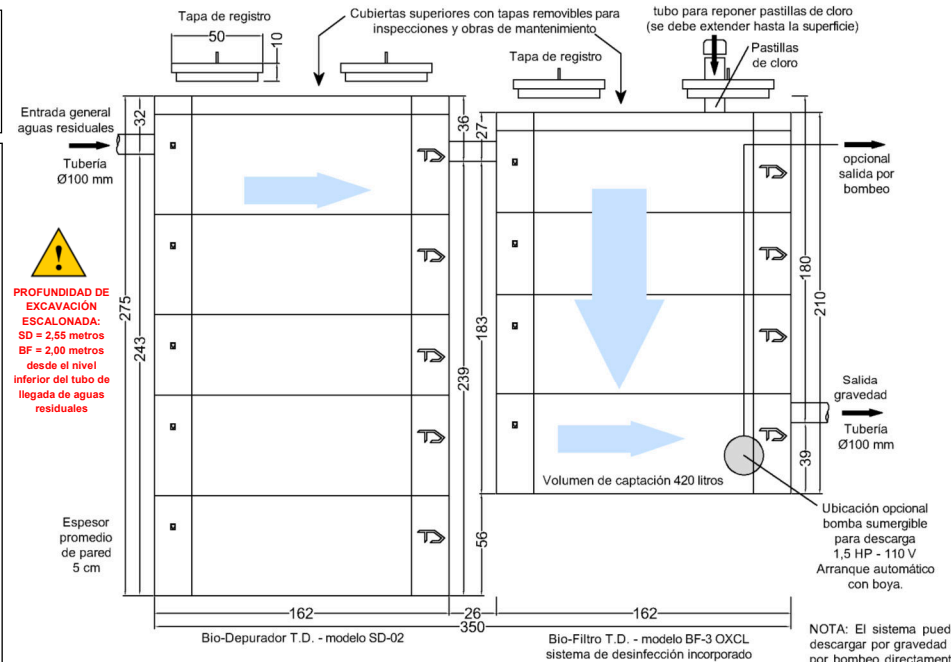
SISTEMA DE TRATAMIENTO TANQUE DIEZ MODELO PTB-OX25 - CAUDAL DIARIO A TRATAR 2,5 M 3 VISTA VERTICAL DE LAS UNIDADES DE TRATAMIENTO - MEDIDAS EN CENTÍMETROS TANQUE DIEZ - DERECHOS RESERVADOS
