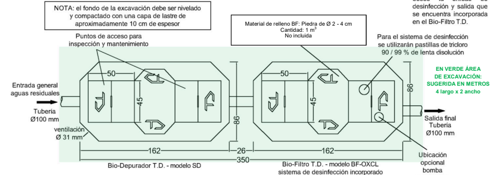
SISTEMA DE TRATAMIENTO TANQUE DIEZ MODELO PTB-OX20 - CAUDAL DIARIO A TRATAR 2 M 3 VISTA SUPERIOR DE LAS UNIDADES DE TRATAMIENTO - MEDIDAS EN CENTÍMETROS TANQUE DIEZ - DERECHOS RESERVADOS
