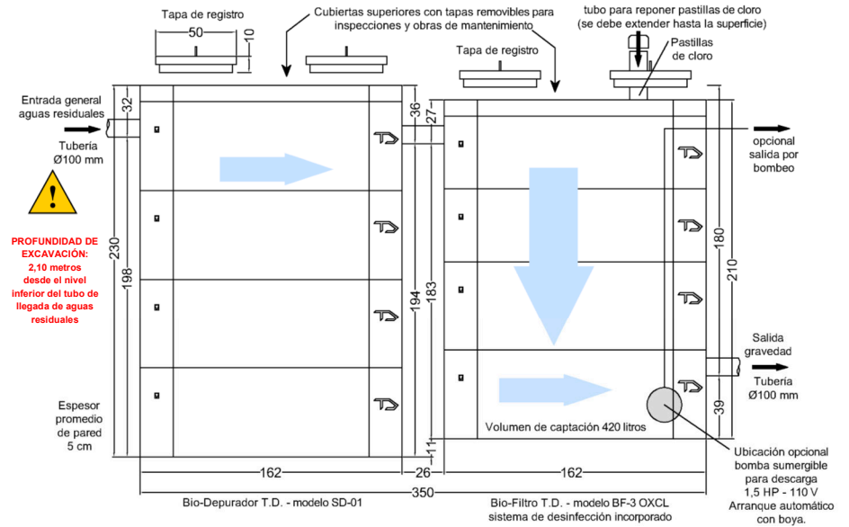
SISTEMA DE TRATAMIENTO TANQUE DIEZ MODELO PTB-OX20 - CAUDAL DIARIO A TRATAR 2 M 3 VISTA VERTICAL DE LAS UNIDADES DE TRATAMIENTO - MEDIDAS EN CENTÍMETROS TANQUE DIEZ - DERECHOS RESERVADOS
