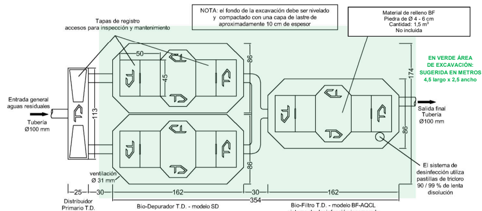
SISTEMA DE TRATAMIENTO TANQUE DIEZ MODELO PTB-AQ40 - CAUDAL DIARIO A TRATAR 4 M 3 VISTA SUPERIOR DE LAS UNIDADES DE TRATAMIENTO - MEDIDAS EN CENTÍMETROS TANQUE DIEZ - DERECHOS RESERVADOS
