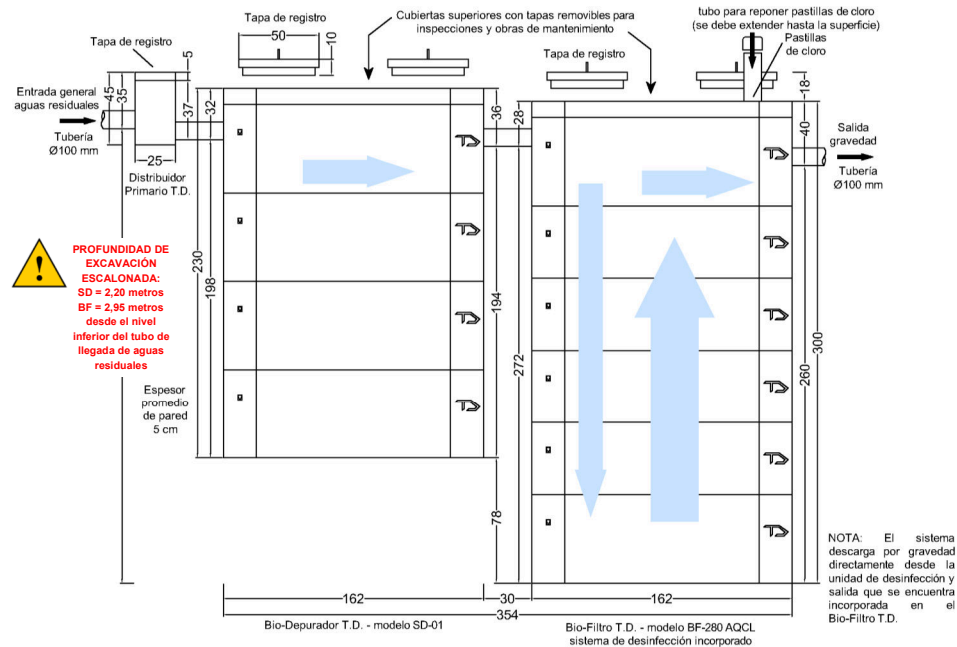
SISTEMA DE TRATAMIENTO TANQUE DIEZ MODELO PTB-AQ40 - CAUDAL DIARIO A TRATAR 4 M 3 VISTA VERTICAL DE LAS UNIDADES DE TRATAMIENTO - MEDIDAS EN CENTÍMETROS TANQUE DIEZ - DERECHOS RESERVADOS
