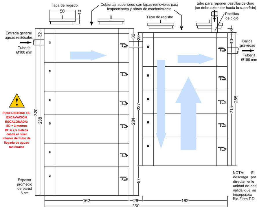
SISTEMA DE TRATAMIENTO TANQUE DIEZ MODELO PTB-AQ30 - CAUDAL DIARIO A TRATAR 3 M 3 VISTA VERTICAL DE LAS UNIDADES DE TRATAMIENTO - MEDIDAS EN CENTÍMETROS TANQUE DIEZ - DERECHOS RESERVADOS
