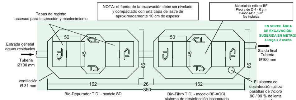
SISTEMA DE TRATAMIENTO TANQUE DIEZ MODELO PTB-AQ30 - CAUDAL DIARIO A TRATAR 3 M 3 VISTA SUPERIOR DE LAS UNIDADES DE TRATAMIENTO - MEDIDAS EN CENTÍMETROS TANQUE DIEZ - DERECHOS RESERVADOS
