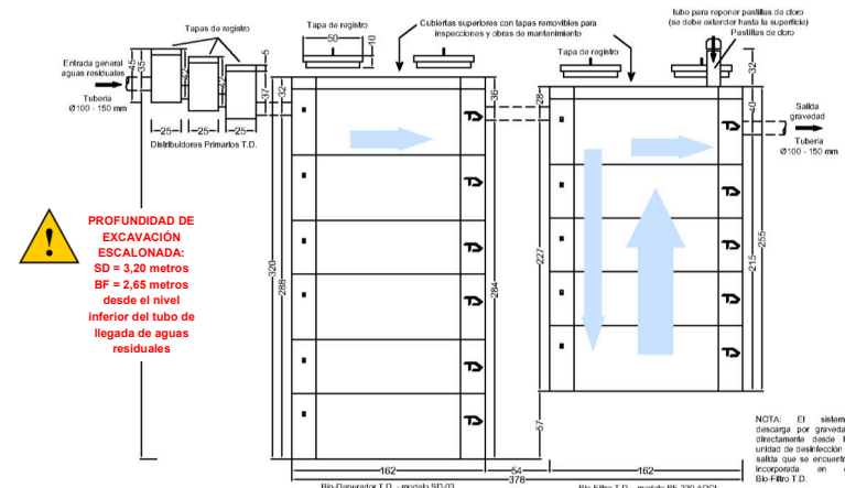
SISTEMA DE TRATAMIENTO TANQUE DIEZ MODELO PTB-AQ240 - CAUDAL DIARIO A TRATAR 24 M 3 VISTA VERTICAL DE LAS UNIDADES DE TRATAMIENTO - MEDIDAS EN CENTÍMETROS TANQUE DIEZ - DERECHOS RESERVADOS
