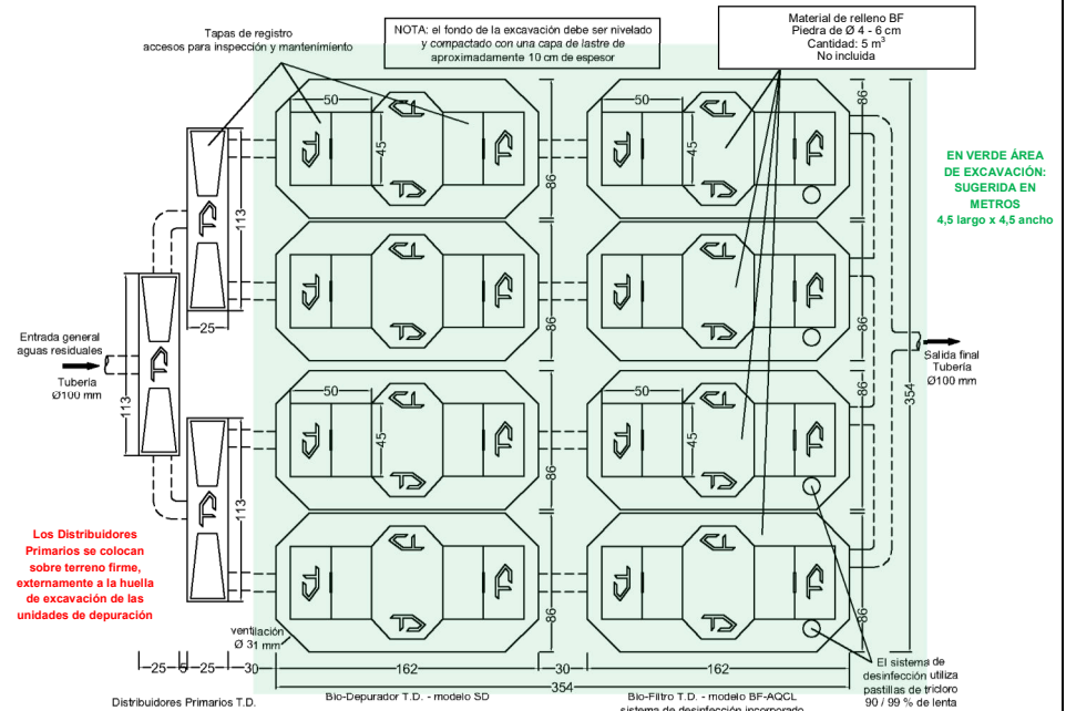
SISTEMA DE TRATAMIENTO TANQUE DIEZ MODELO PTB-AQ140 - CAUDAL DIARIO A TRATAR 14 M 3 VISTA SUPERIOR DE LAS UNIDADES DE TRATAMIENTO - MEDIDAS EN CENTÍMETROS TANQUE DIEZ - DERECHOS RESERVADOS
