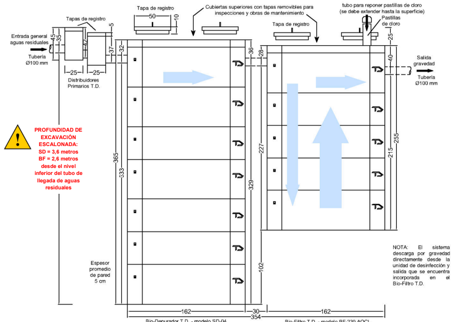
SISTEMA DE TRATAMIENTO TANQUE DIEZ MODELO PTB-AQ140 - CAUDAL DIARIO A TRATAR 14 M 3 VISTA VERTICAL DE LAS UNIDADES DE TRATAMIENTO - MEDIDAS EN CENTÍMETROS TANQUE DIEZ - DERECHOS RESERVADOS
