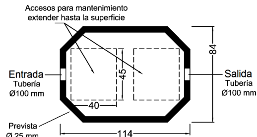
Unidad de Captación T.D. Modelo KMC-F sección horizontal - medidas en cm ©TANQUE DIEZ - Derechos Reservados
