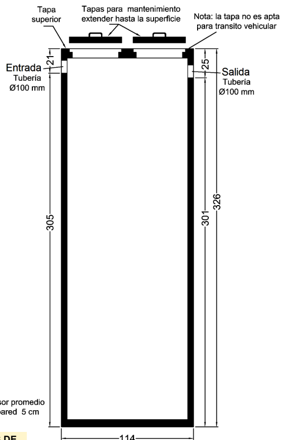
Unidad de Captación T.D. Modelo KMC-F sección vertical - medidas en cm ©TANQUE DIEZ - Derechos Reservados
