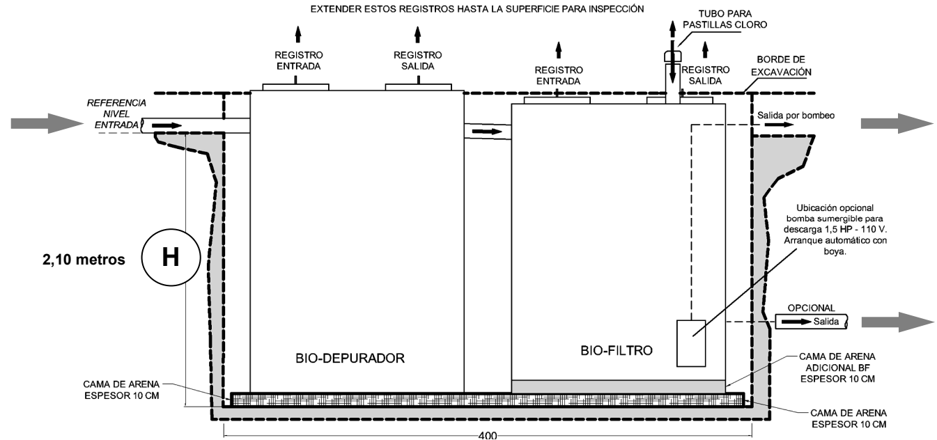
SISTEMA TANQUE DIEZ MODELO BPR-OX01 - VISTA VERTICAL PARA EXCAVACIÓN (LINEAL) MEDIDAS EN CENTIMETROS - TANQUE DIEZ - DERECHOS RESERVADOS
