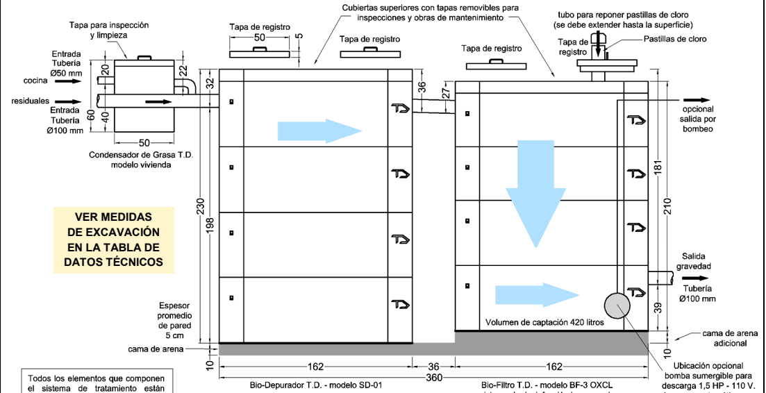
SISTEMA BPR TANQUE DIEZ MODELO BPR-OX01 - CAUDAL DIARIO A TRATAR 2 M 3 UNIDADES DE DEPURACIÓN - VISTA VERTICAL - MEDIDAS EN CENTÍMETROS TANQUE DIEZ - DERECHOS RESERVADOS
