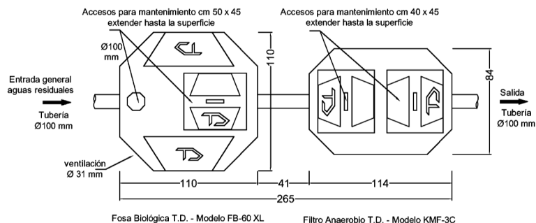
SISTEMA BIOLÓGICO MEJORADO TANQUE DIEZ - MODELO SBM-3000 CAUDAL DIARIO APLICABLE 3 M 3 - VISTA SUPERIOR - MEDIDAS EN CENTÍMETROS TANQUE DIEZ - DERECHOS RESERVADOS
