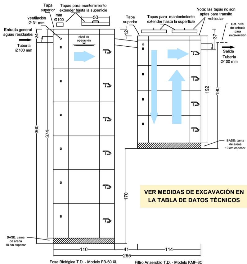
SISTEMA BIOLÓGICO MEJORADO TANQUE DIEZ - MODELO SBM-3000 CAUDAL DIARIO APLICABLE 3 M 3 - VISTA VERTICAL - MEDIDAS EN CENTÍMETROS TANQUE DIEZ - DERECHOS RESERVADOS
