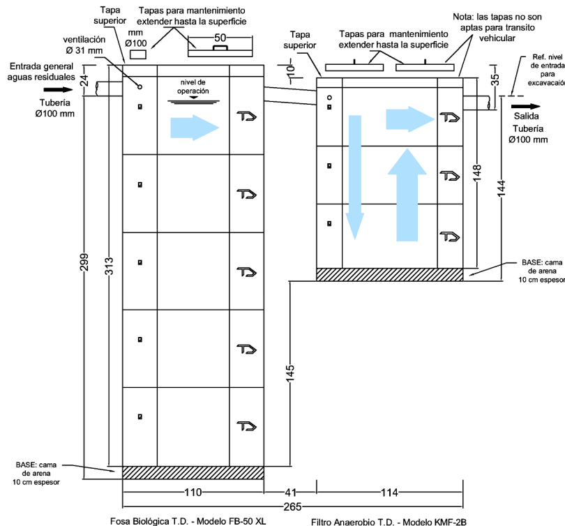
Fosa Biológica T.D. - Modelo FB-50 XL Filtro Anaerobio T.D. - Modelo KMF-2B
