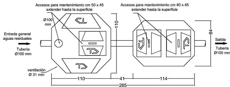
Fosa Biológica T.D. - Modelo FB-50 XL Filtro Anaerobio T.D. - Modelo KMF-2B
