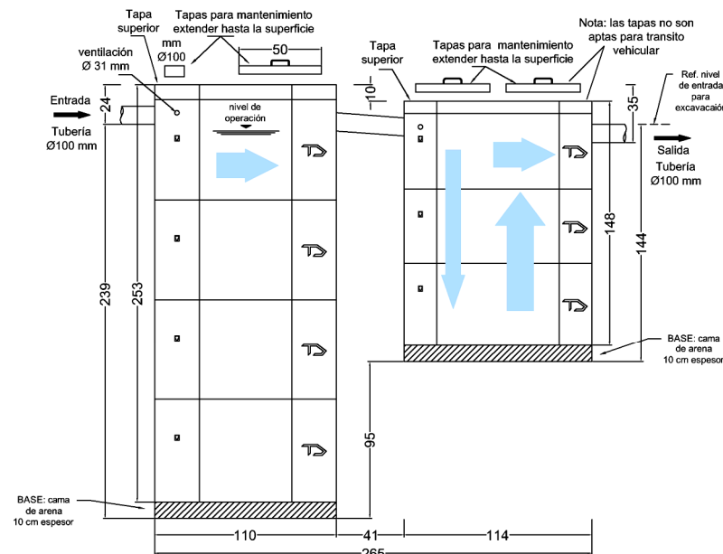
Fosa Biológica T.D. - Modelo FB-40 XL Filtro Anaerobio T.D. - Modelo KMF-2B
