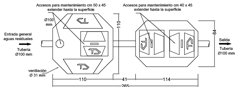
Fosa Biológica T.D. - Modelo FB-40 XL Filtro Anaerobio T.D. - Modelo KMF-2B
