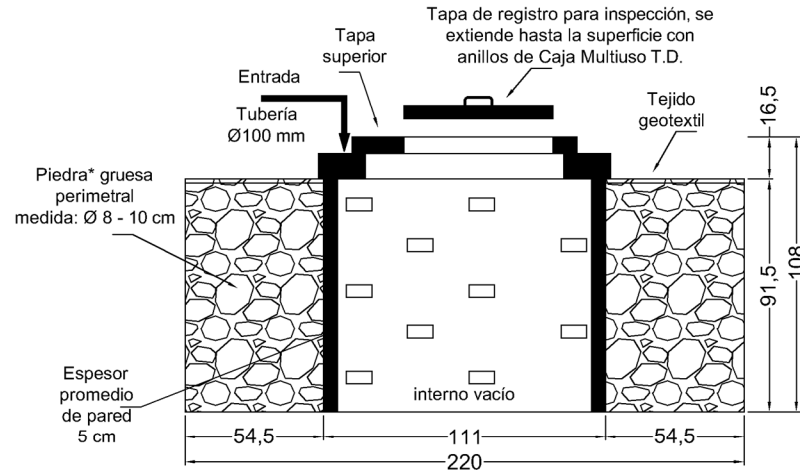
Pozo Absorbente Prefabricado T.D. Modelo PAP-4 con piedra perimetral sección vertical - medidas en cm
