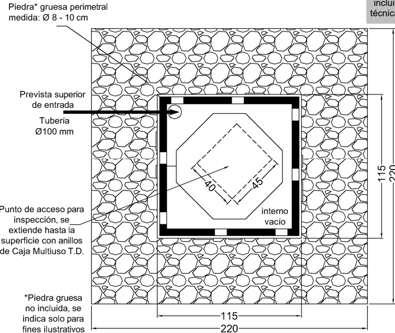
Pozo Absorbente Prefabricado T.D. Modelo PAP-4 con piedra perimetral sección horizontal - medidas en cm
