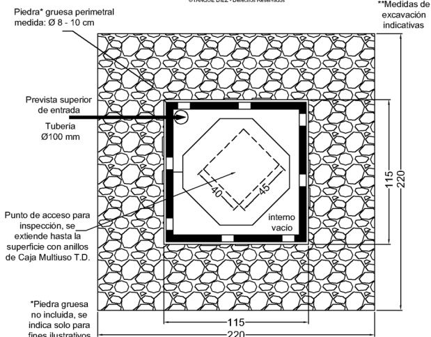
Pozo Absorbente Prefabricado T.D. Modelo PAP-12 con piedra perimetral sección horizontal - medidas en cm ©TANQUE DIEZ - Derechos Reservados
