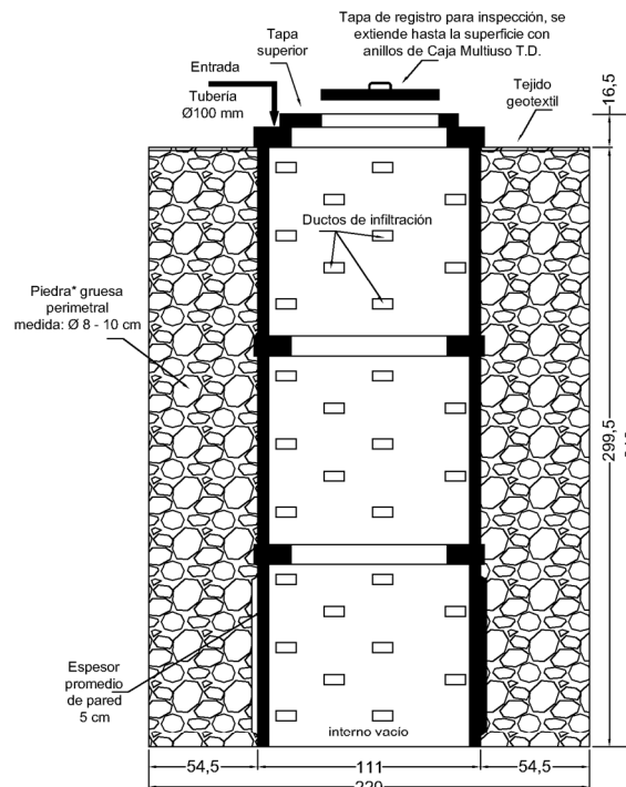
Pozo Absorbente Prefabricado T.D. Modelo PAP-12 con piedra perimetral sección vertical - medidas en cm ©TANQUE DIEZ - Derechos Reservados
