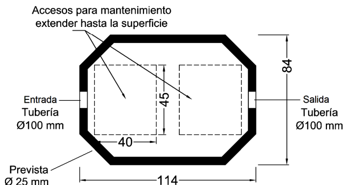
Unidad de Captación T.D. Modelo KMC-B sección horizontal - medidas en cm ©TANQUE DIEZ - Derechos Reservados
