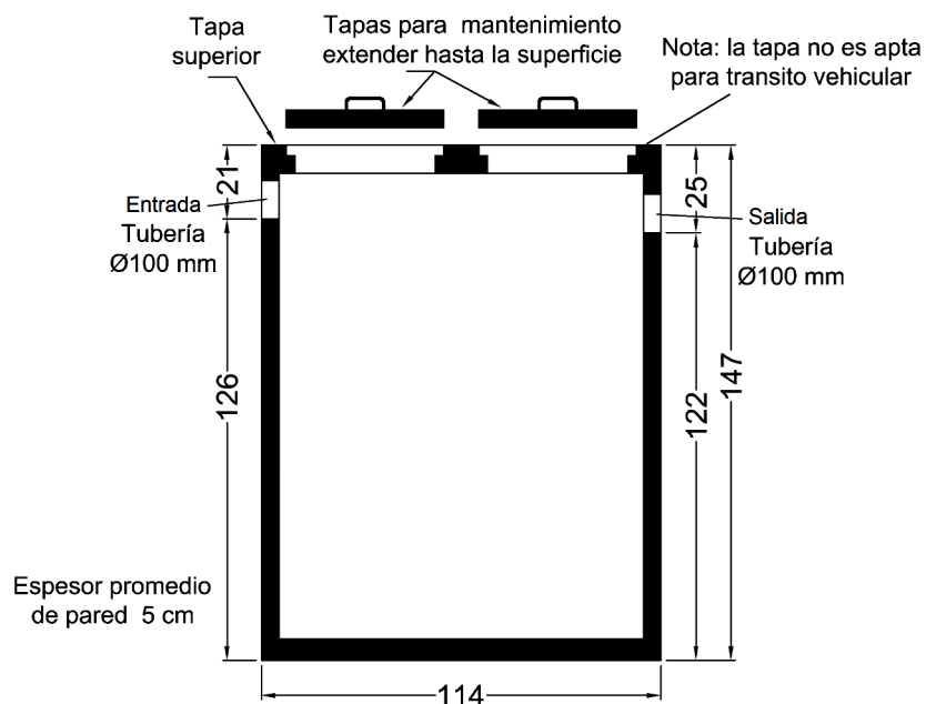
Unidad de Captación T.D. Modelo KMC-B sección vertical - medidas en cm ©TANQUE DIEZ - Derechos Reservados
