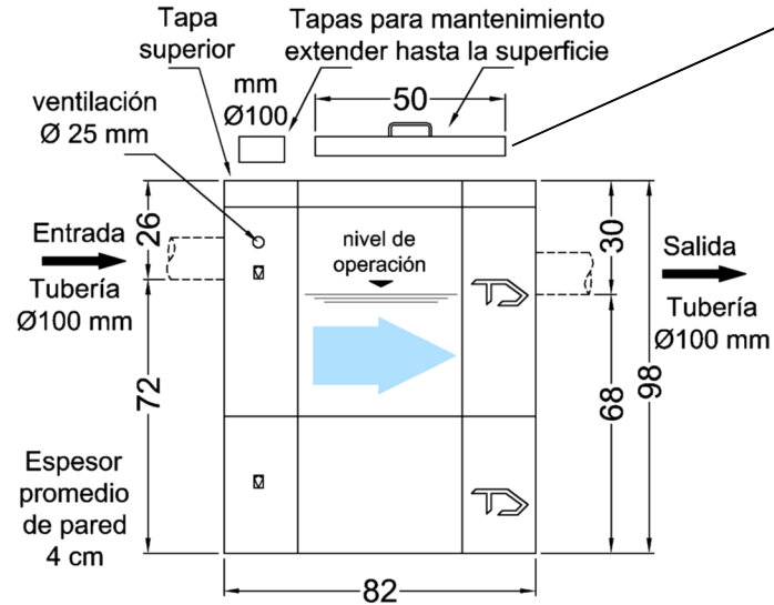
Fosa Biológica T.D. Modelo FB-3 vista vertical - medidas en cm ©TANQUE DIEZ - Derechos Reservados
