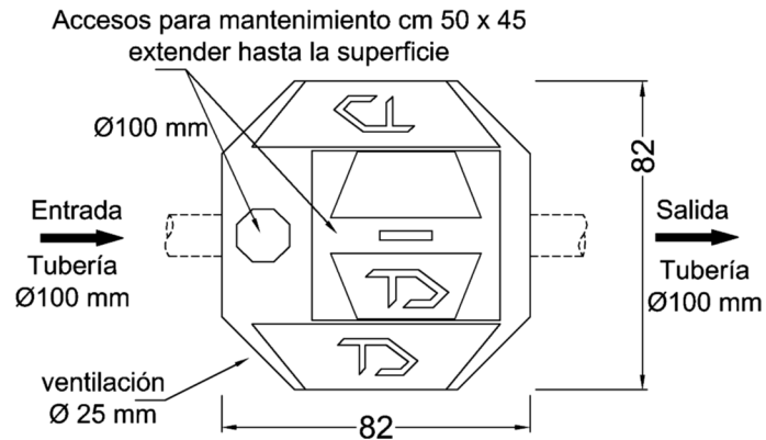
Fosa Biológica T.D. Modelo FB-3 vista superior - medidas en cm ©TANQUE DIEZ - Derechos Reservados
