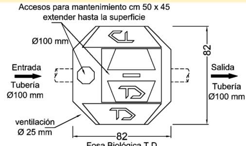
Fosa Biológica T.D. Modelo FB-20 vista superior - medidas en cm ©TANQUE DIEZ - Derechos Reservados
