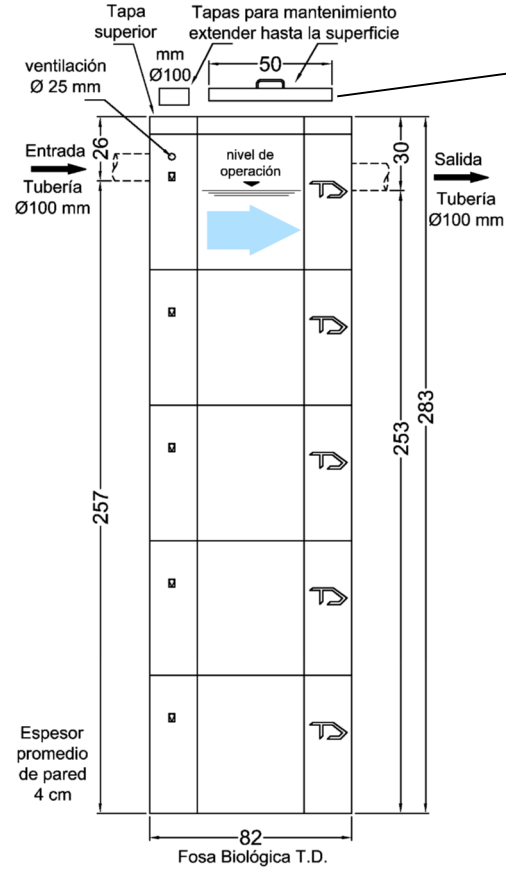
Fosa Biológica T.D. Modelo FB-20 vista vertical - medidas en cm ©TANQUE DIEZ - Derechos Reservados
