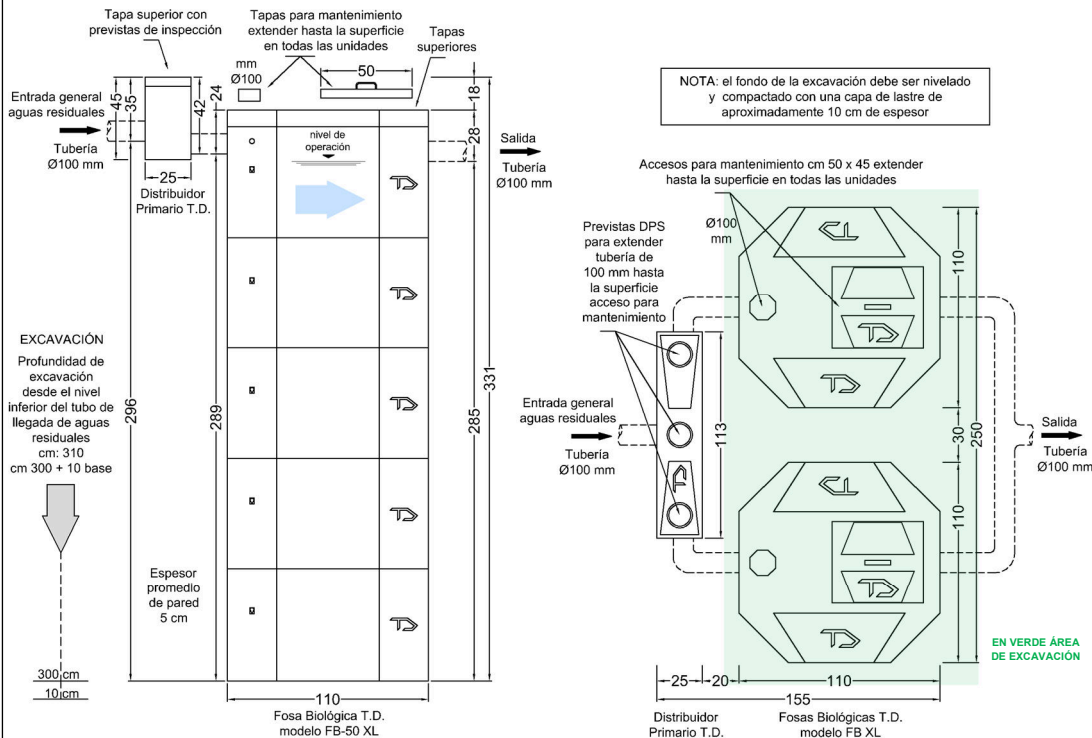
SISTEMA FB-100XL COMPUESTO POR 2 UNIDADES DE FOSAS BIOLÓGICAS TANQUE DIEZ CAUDAL MÁXIMO DIARIO A TRATAR 5 M 3 VISTA VERTICAL DE LAS UNIDADES DE TRATAMIENTO MEDIDAS EN CENTÍMETROS TANQUE DIEZ - DERECHOS RESERVADOS
